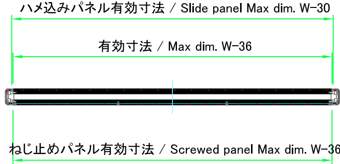
A-A ( 1 : 9 )
